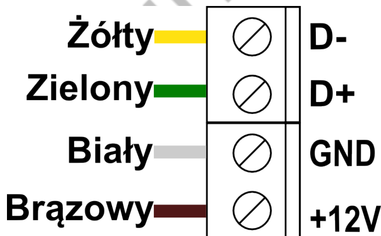
Ilustracja 1: Podłączenie panelu
